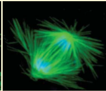
Anafase
